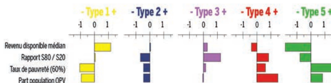
Distance de la moyenne de chaque type à la moyenne générale des agglomérations observées
